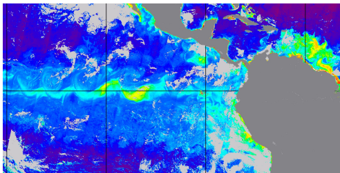
Divergence équatoriale
